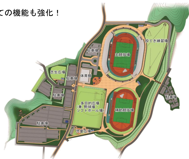
【山之口運動公園施設配置計画（案）】 宮崎県策定『県陸上競技場整備基本計画』より
