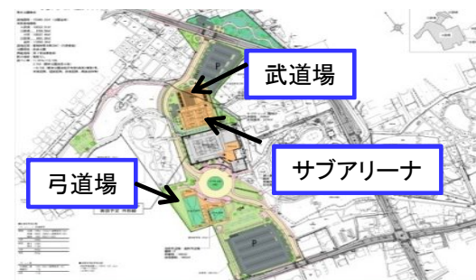
計画配置図
