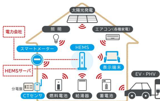
図 HEMS の導入イメージ
